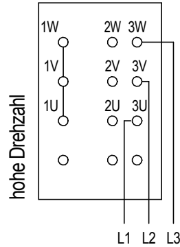
YY-Schaltung Wicklung 1
