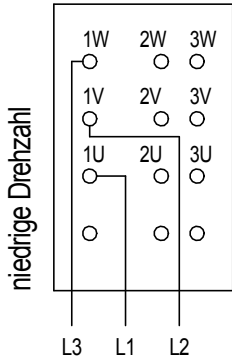
Y-Schaltung Wicklung 1
