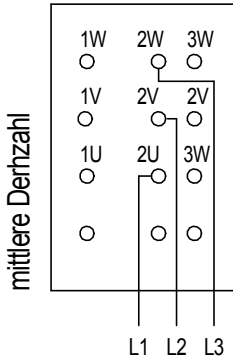
Y-Schaltung Wicklung 2
