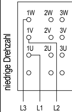
Y-Schaltung Wicklung 1
