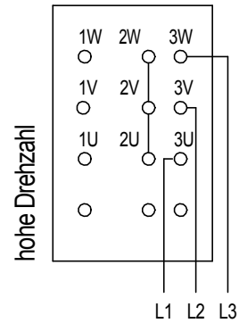
YY-Schaltung Wicklung 2
