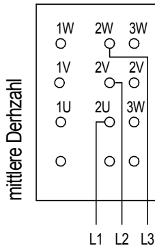
\Delta -Schaltung Wicklung 2
